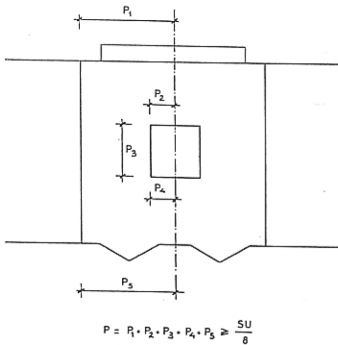
Fig. 11 – Perímetre de tancament (art. 31.1.)
