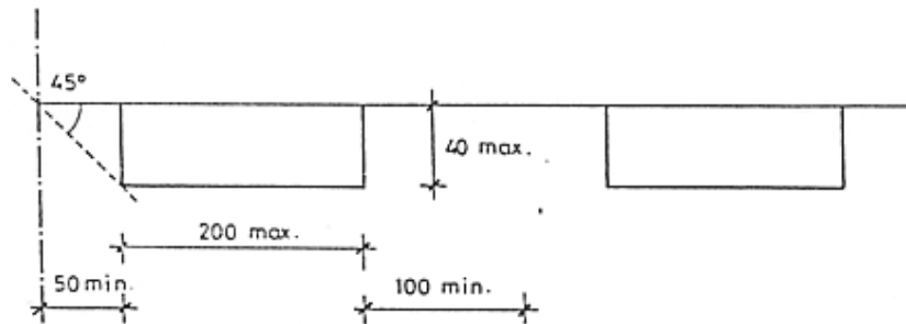
Fig. 4 – Vol en carrer d'ample < o = a 6 m. (art. 4.)
