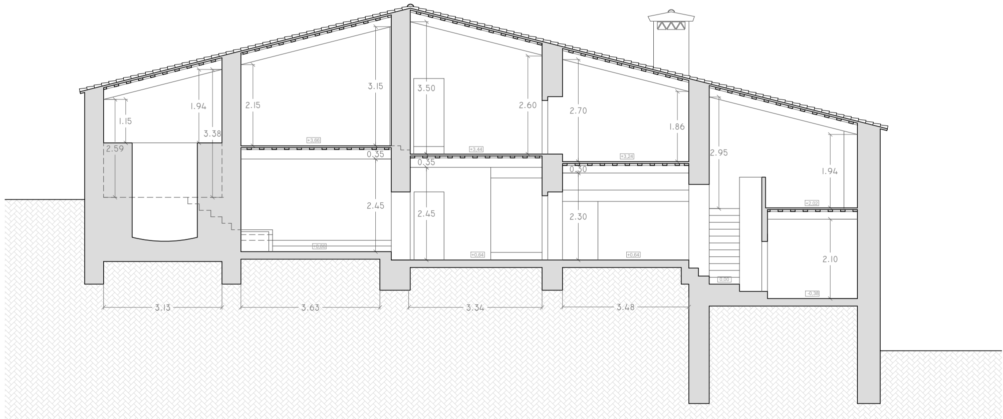
SECCIÓ A-A'
