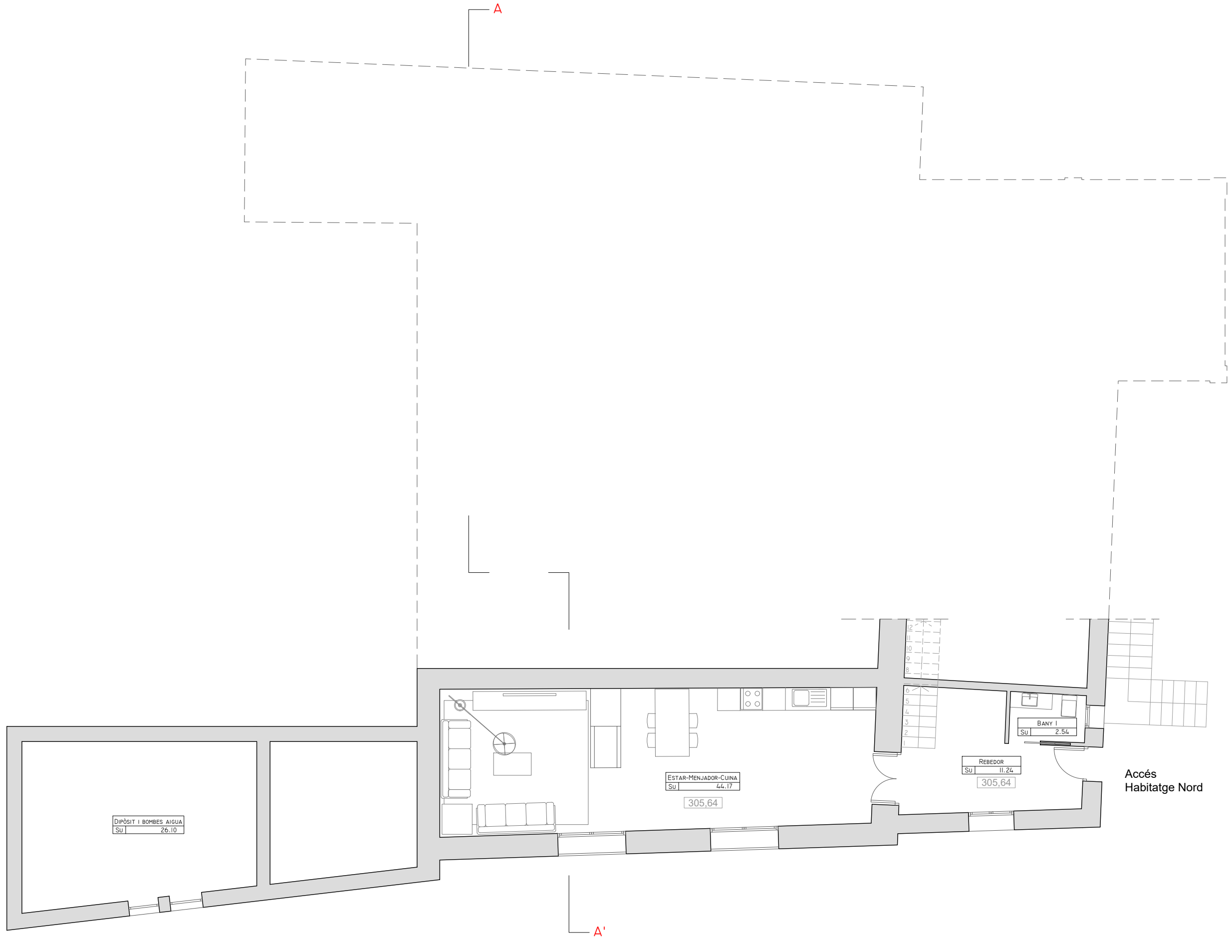
PLANTA COTA 305,64
