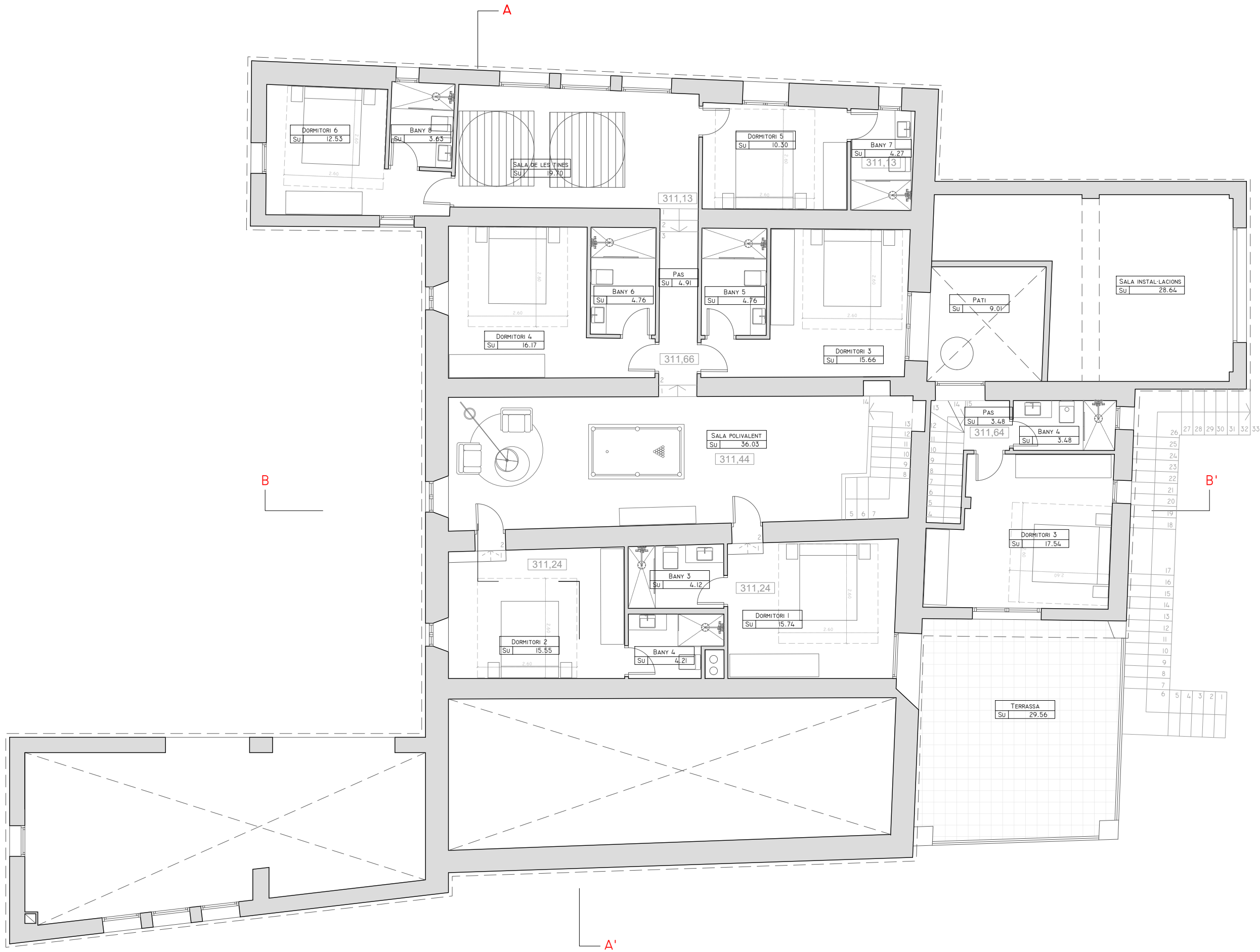
PLANTA COTA 311,44
