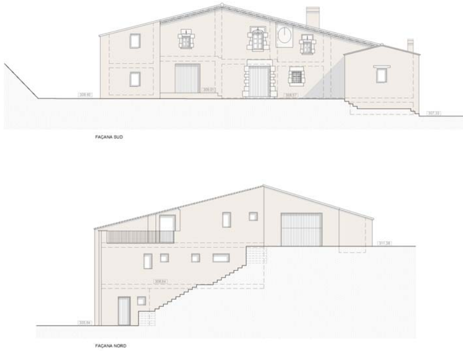
Façanes Sud i Nord
