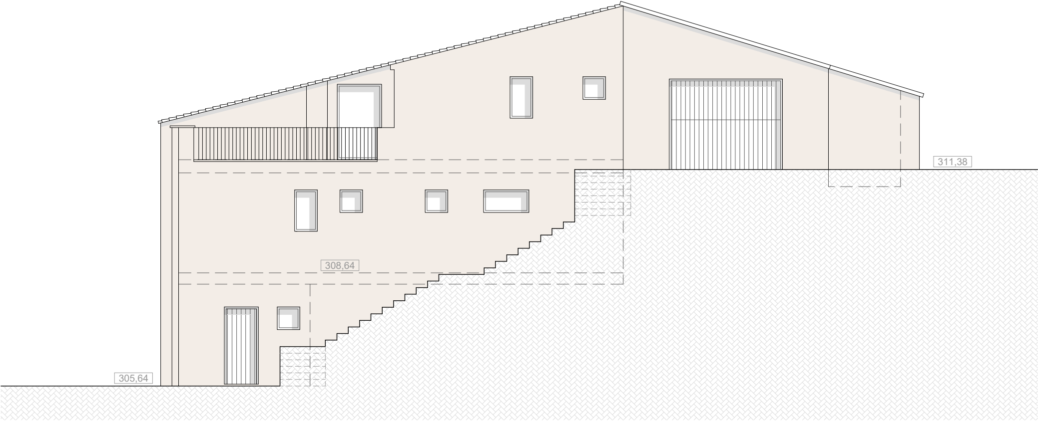
FAÇANA NORD
