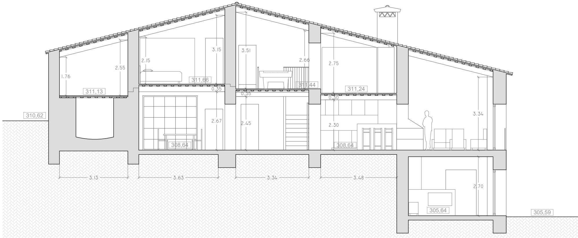
SECCIÓ A-A'
