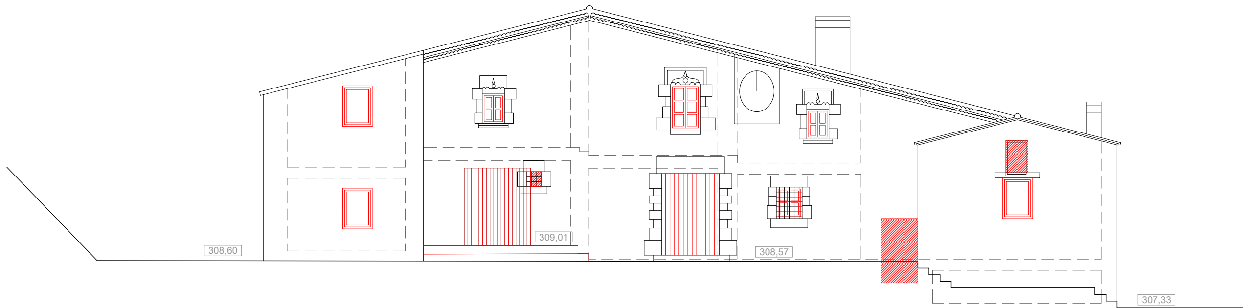
FAÇANA SUD
