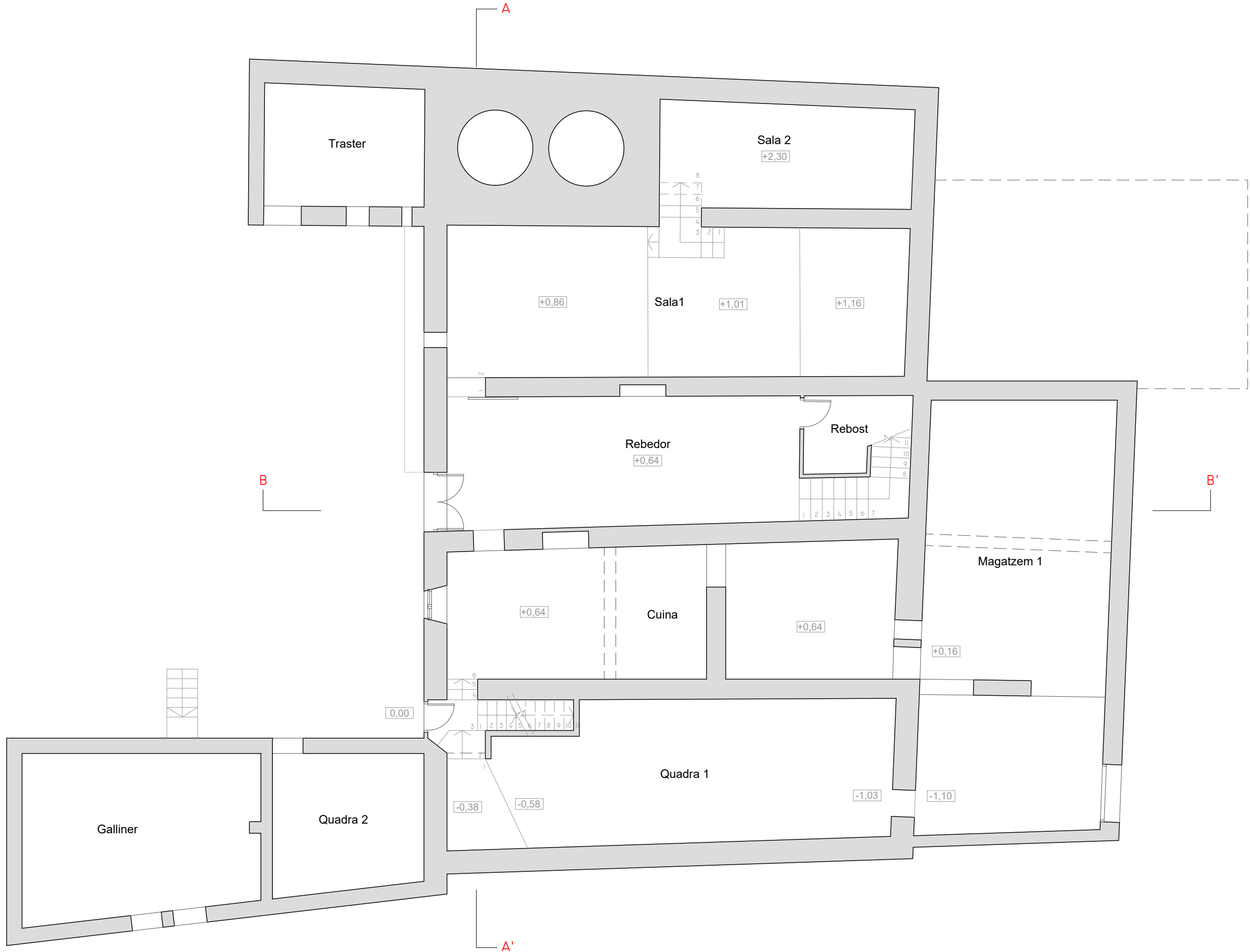
PLANTA COTA 308,64
