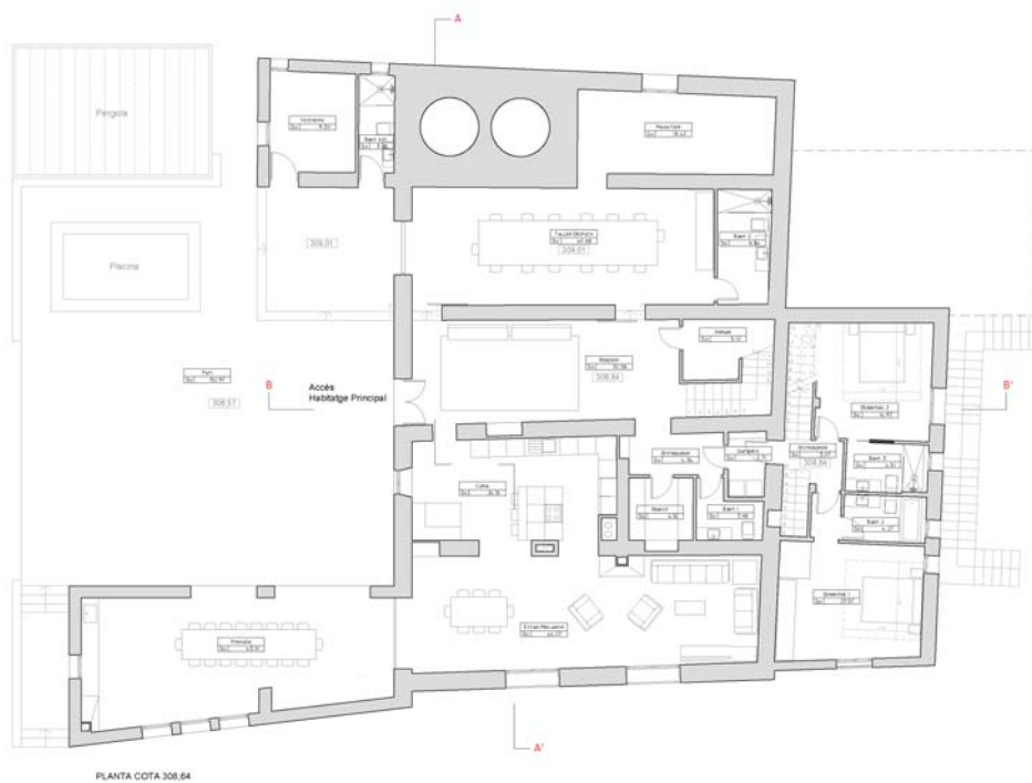
Planta cota 308,64
