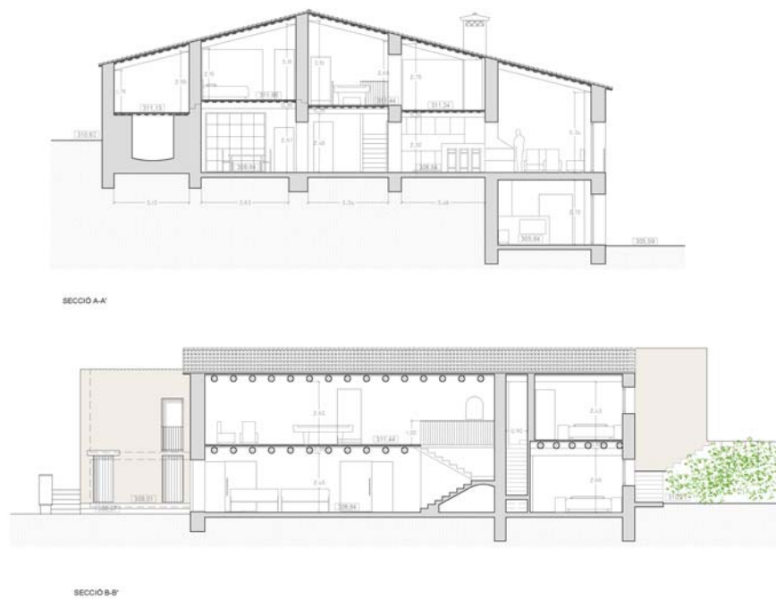
Secció A-A' i B-B'
